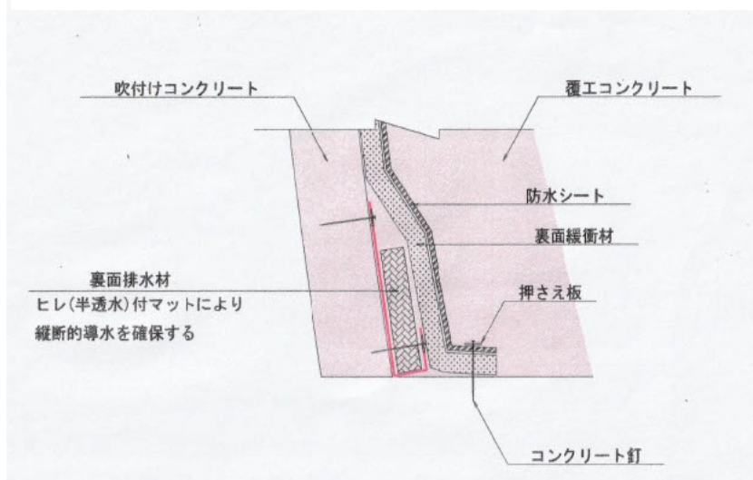
裏面排水設置図面
