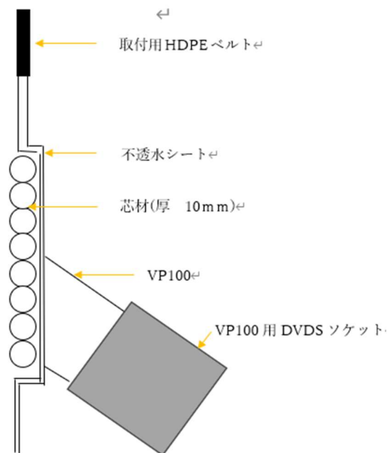
構造図
